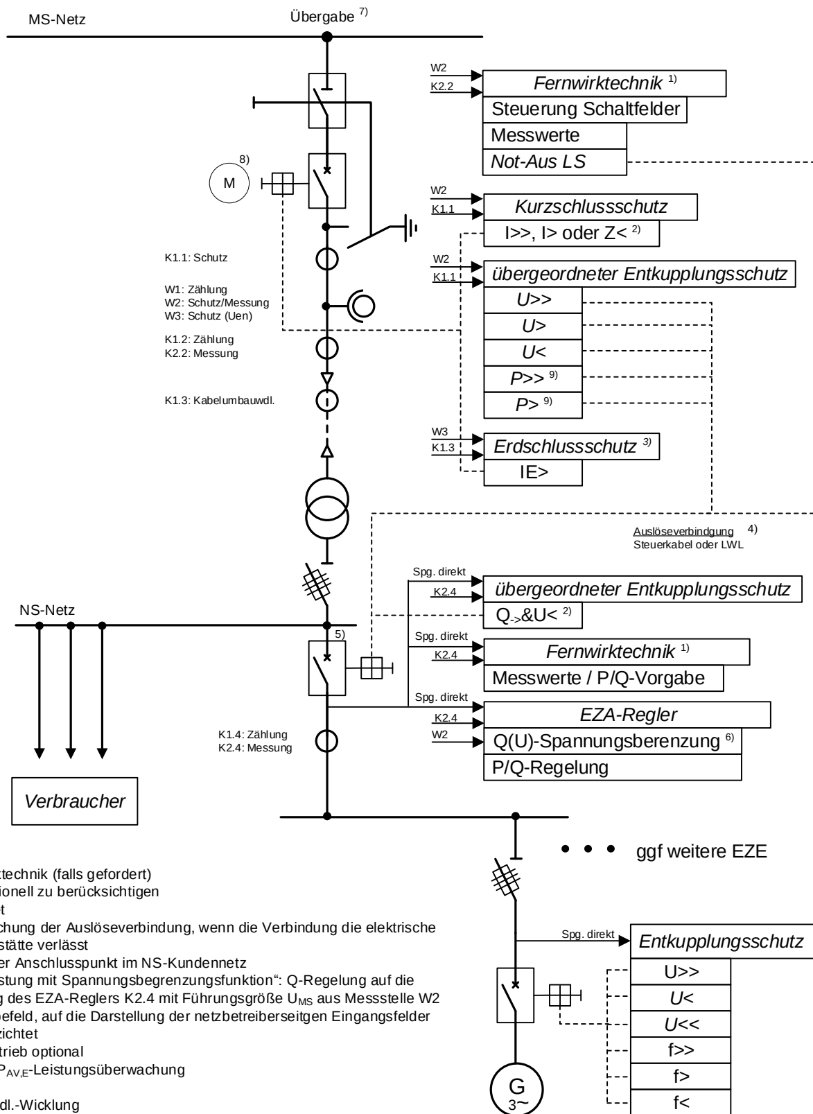
Bild 8- Mischanlage – Beispiel für eine an das Mittelspannungsnetz angeschlossenen Kundenanlage mit Bezug und Erzeugungsanlage mit Leistungsschalter und einer Erzeugungseinheit ohne Inselbetriebsmöglichkeit (Anschluss nicht in UW bzw. Schaltstation)
